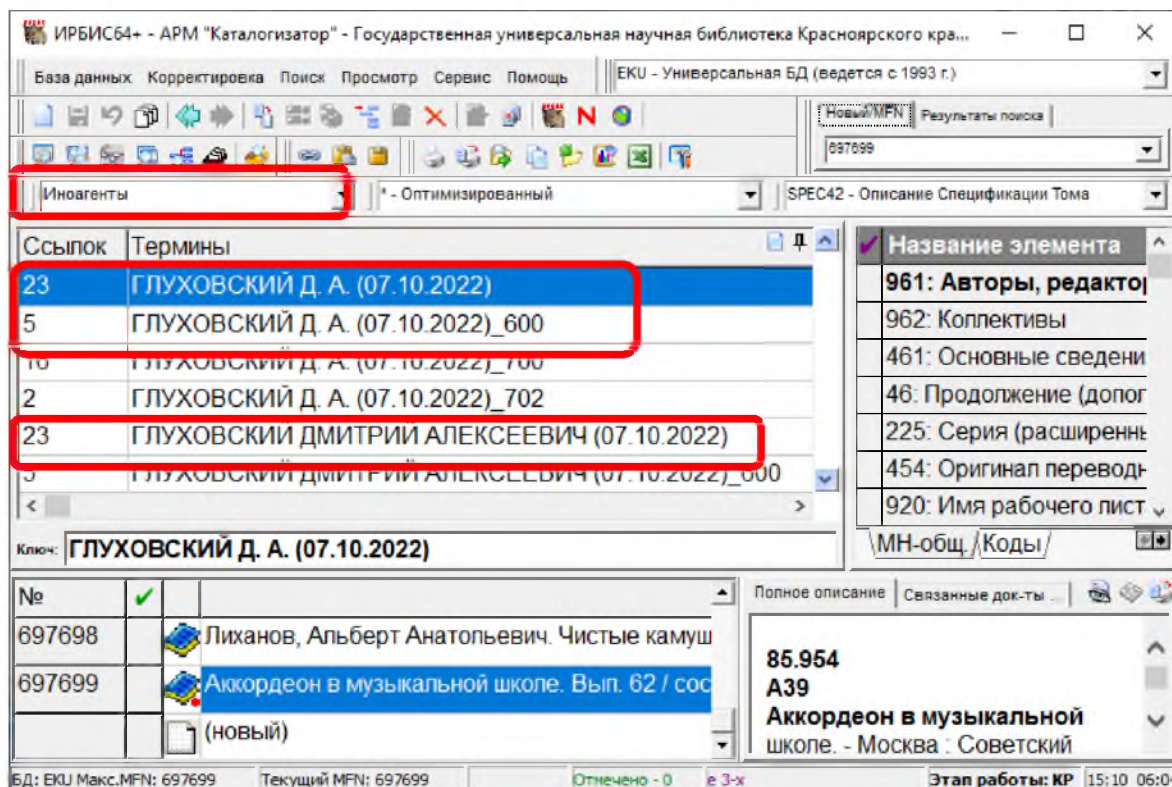
Рис. 10. Поиск "Иноагенты"
