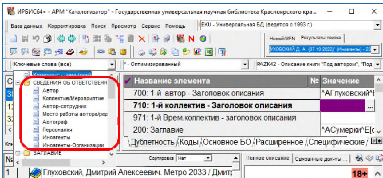
Рис. 9. Поиск «Иноагенты»
